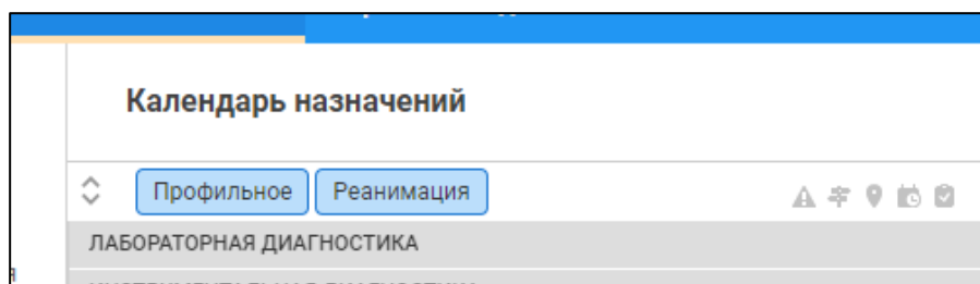
Рисунок 8 - Фильтр назначений
