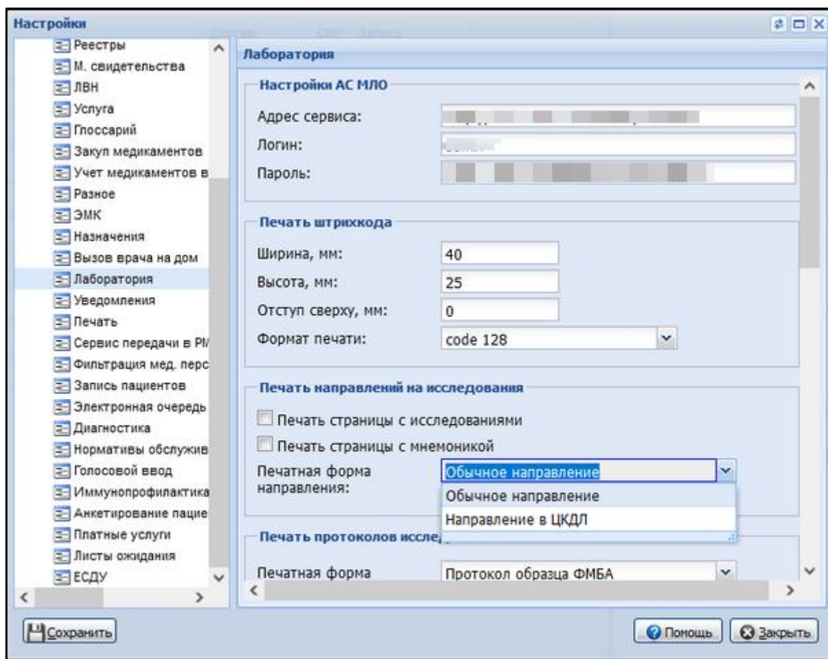
Рисунок 34 - Настройки печати
